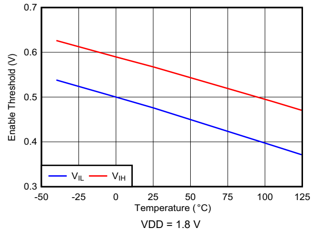
图 6-4. EN Threshold vs Temperature V_{DD} = 1.8\text{ V}
